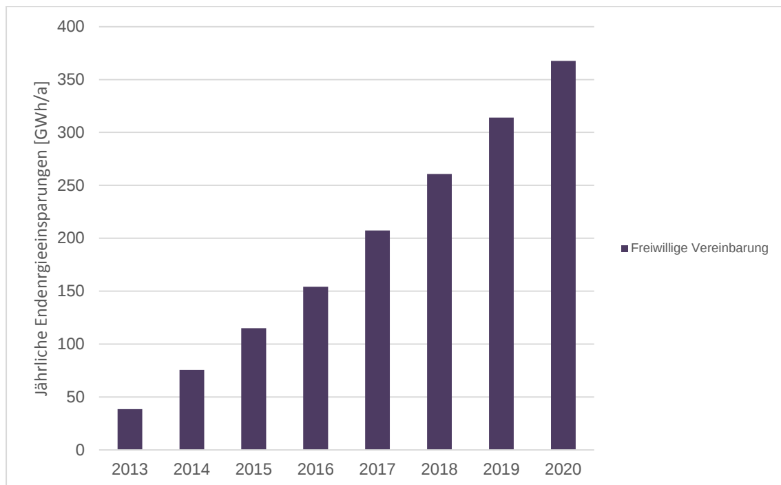
Abbildung 4: Realisierte Endenergieeinsparungen in den Jahren 2013-2015, sowie die erwartete Entwicklung der Endenergieeinsparungen durch die freiwillige Vereinbarung mit der Industrie in den Jahren 2016-2020.
