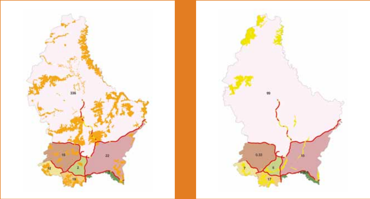
Schéma 30: Superposition des zones du réseau Natura 2000 sur la carte des espaces non fragmentées par des autoroutes. A gauche: zones spéciales de conservation (zones habitats). A droite: zones de protection spéciale (zones oiseaux). Surface en km². Fond de carte: © Administration du Cadastre et de la Topographie - Tous droits réservés à l'Etat du Grand-Duché de Luxembourg.
