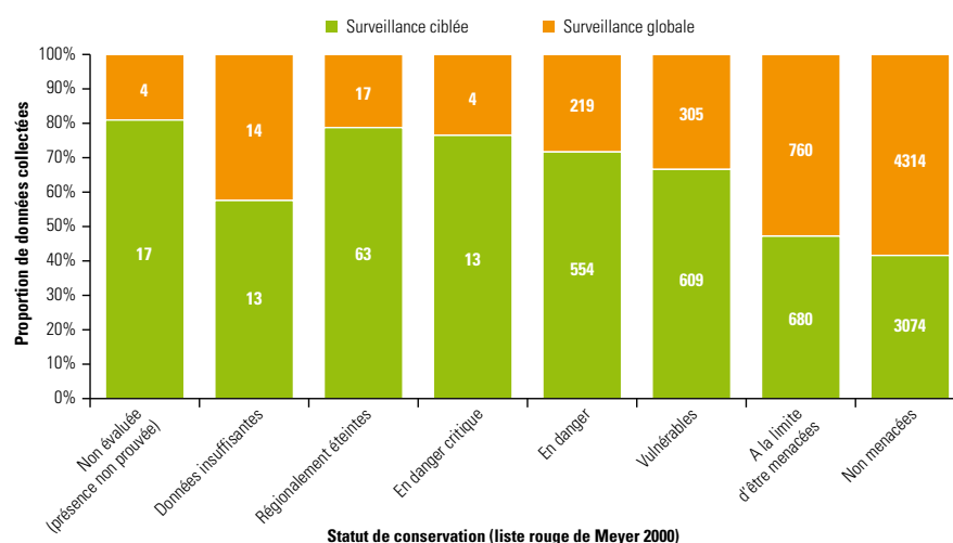
Figure 3. Répartition par statut de conservation (liste rouge de Meyer 2000) des données relatives aux papillons de jours collectées lors des programmes de surveillance globale et ciblée en 2011. Le nombre de données est indiqué pour chaque statut et chaque programme de surveillance.
