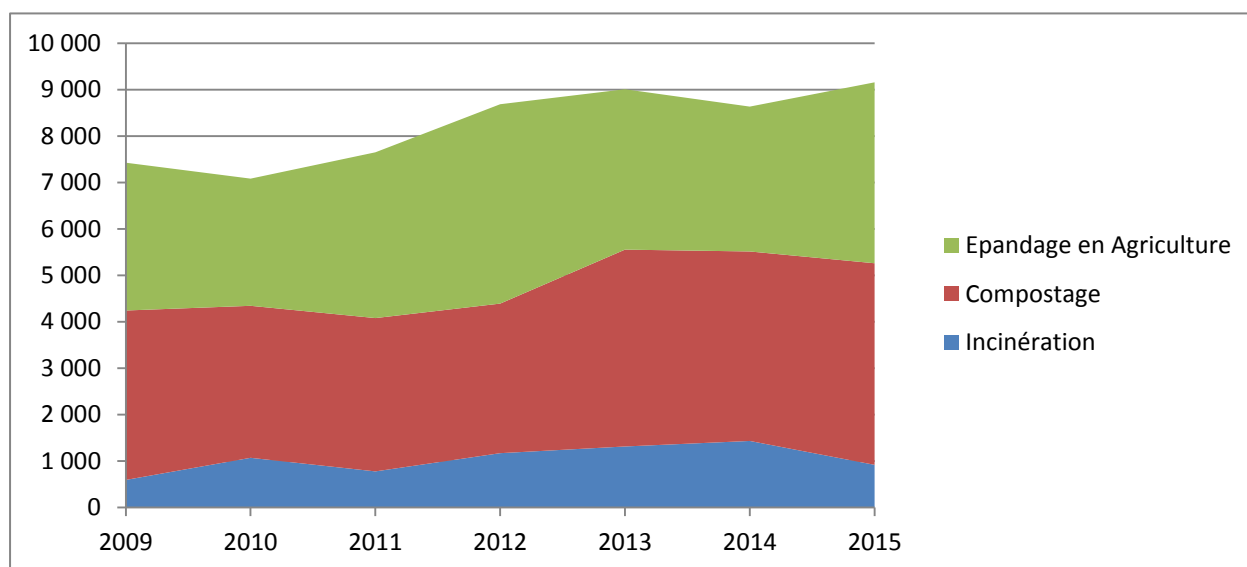
FIGURE 52: FILIERES D'ELIMINATION ET DE VALORISATION DES BOUES D'EPURATION EXPRIMEES EN MG DE MATIERE SECHE (2009-2015)
