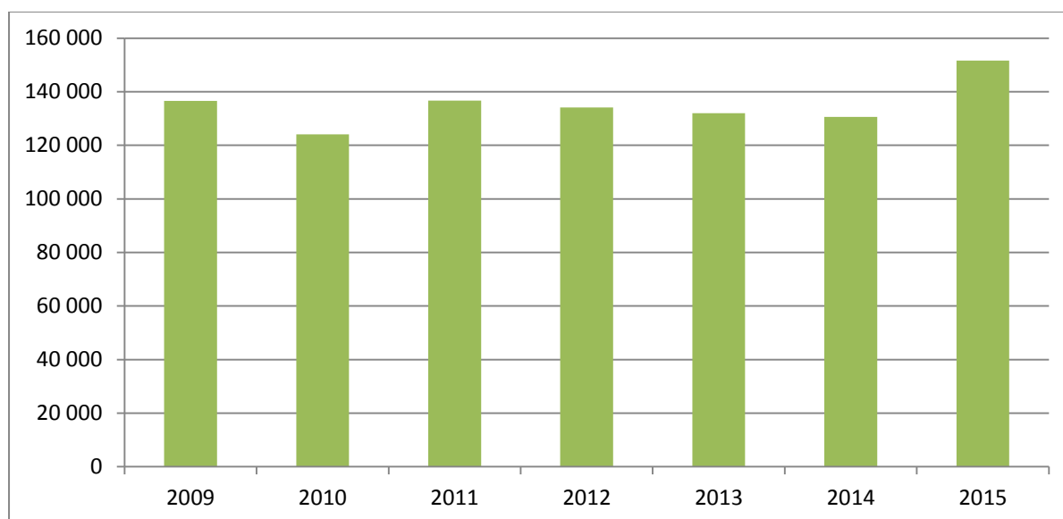
FIGURE 11: EVOLUTION DES QUANTITES DE DECHETS TRAITEES DANS L'INSTALLATION D'INCINERATION DU SIDOR (2009-2015) (EXPRIMEES EN MG)
